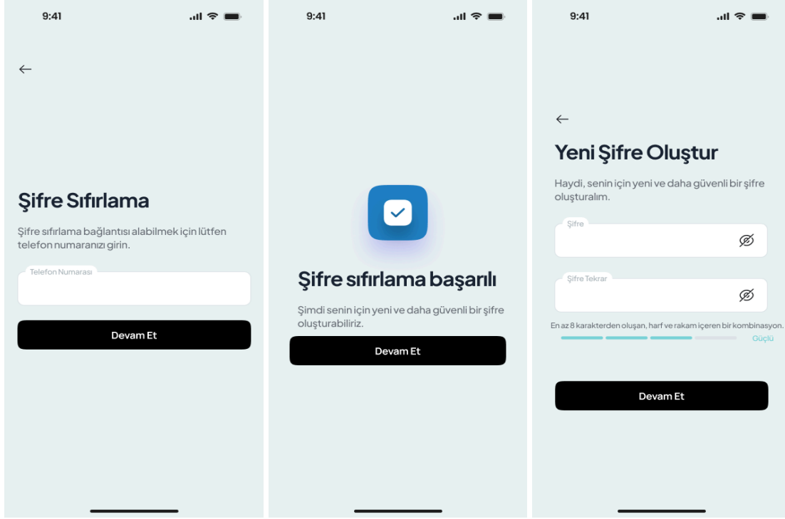
Görsel 2.2: Mobil Uygulama Şifre Sıfırlama Ekranları
